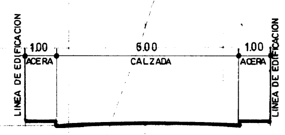
SECCION TIPO DE VIARIO PROYECTADO
